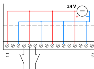
Aktivní režim (pro pasivní čidla)
