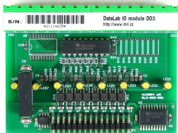
Modul DataLab DO3
