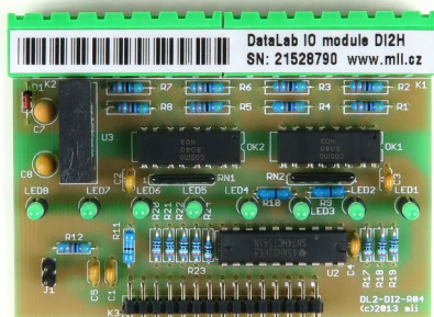
Modul DataLab DI2
