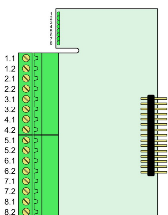
Označení svorek
