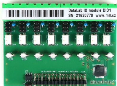
Modul DataLab DIO1
