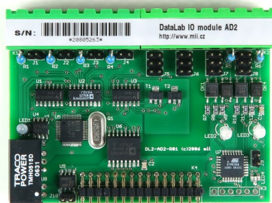
Modul DataLab AD2
